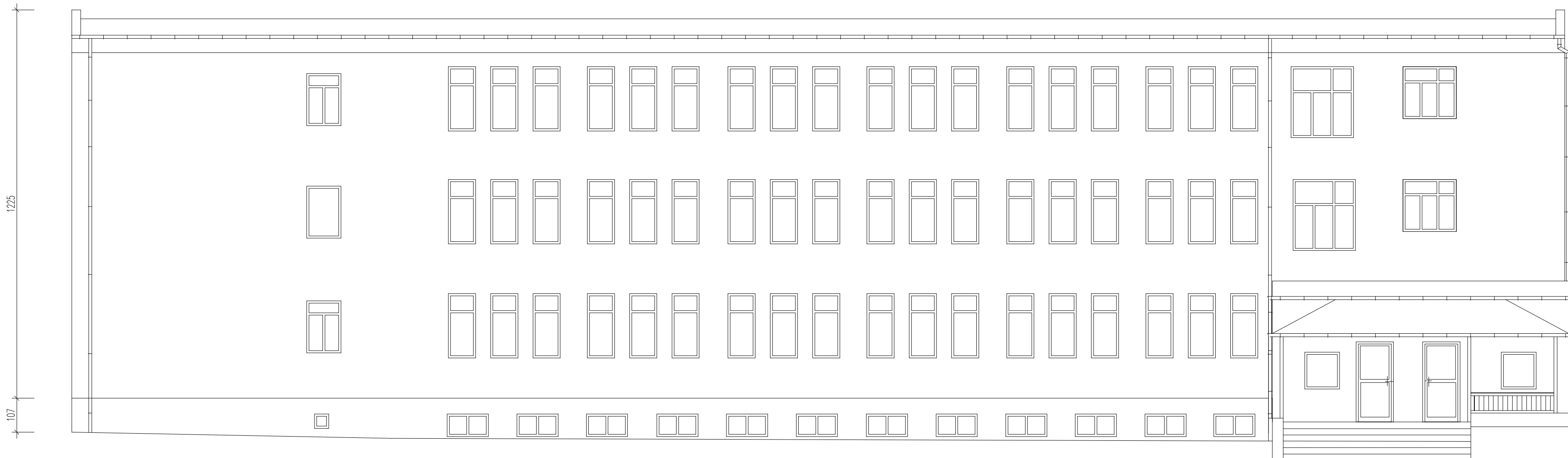
ELEWACJA "B"
