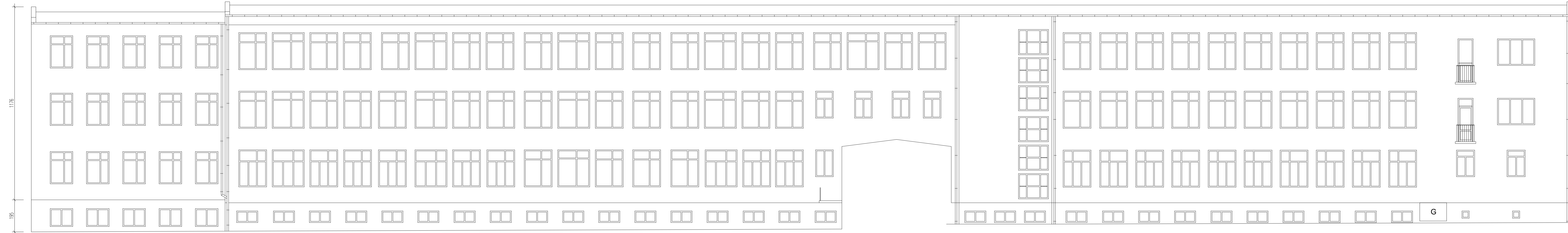
ELEWACJA "L"
